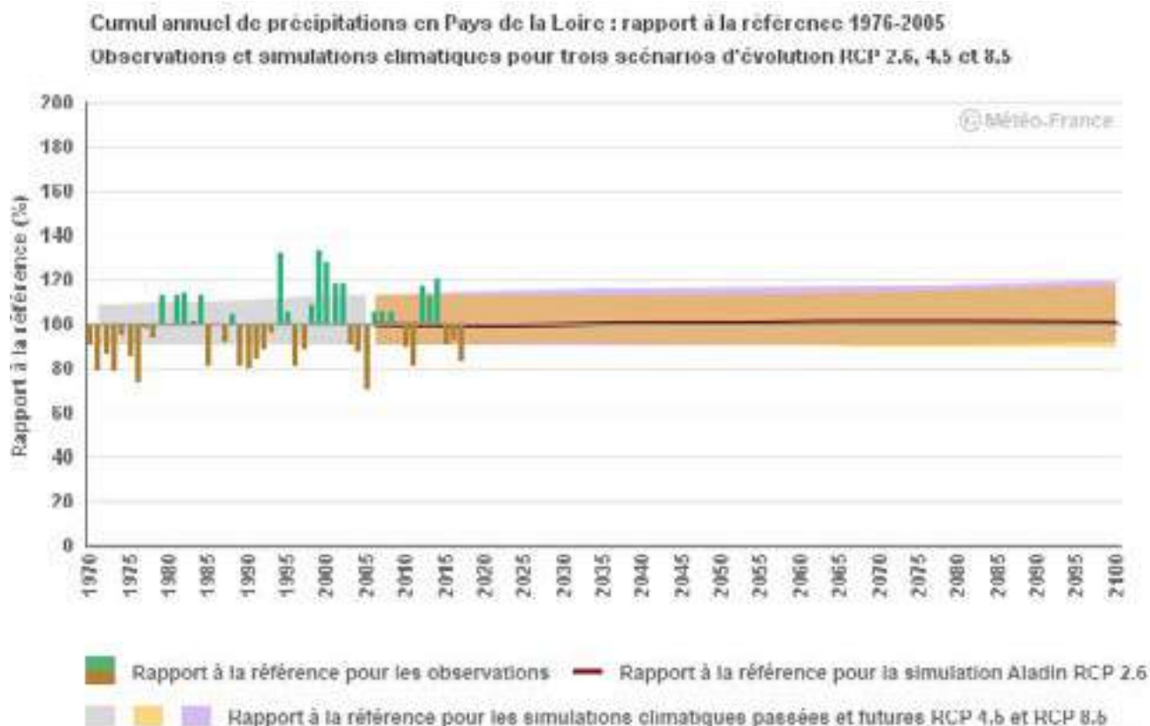
Illustration 27 : cumul annuel de précipitation en Pays de la Loire et projection climatique. Source : Climat HD Météo France
