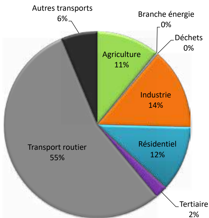
Profil d'émissions de l'oxyde d'Azote 2016
