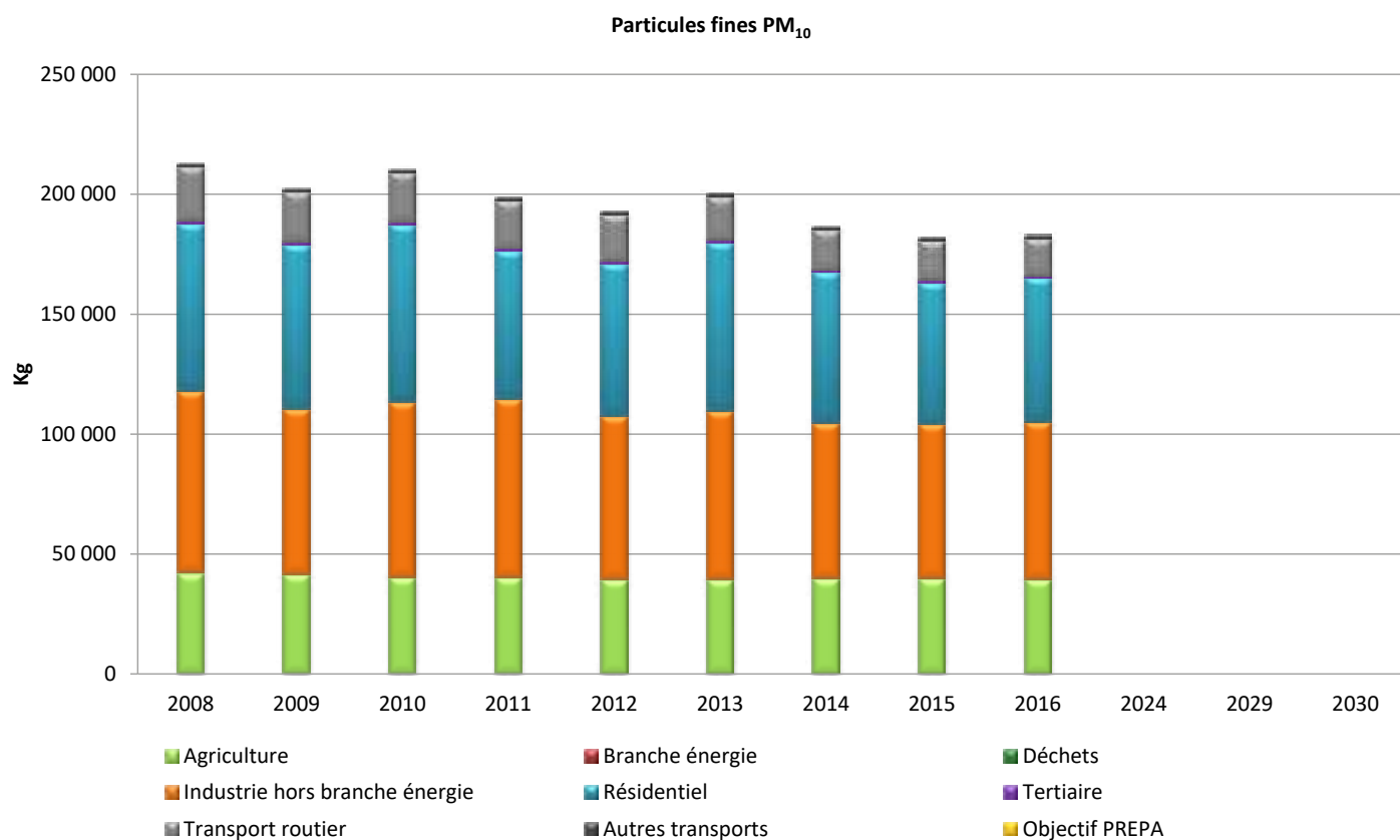
Graphique 43 : évolution des émissions de particules fines 10 par secteur. Source : données Air Pays de la Loire 2008-2016
