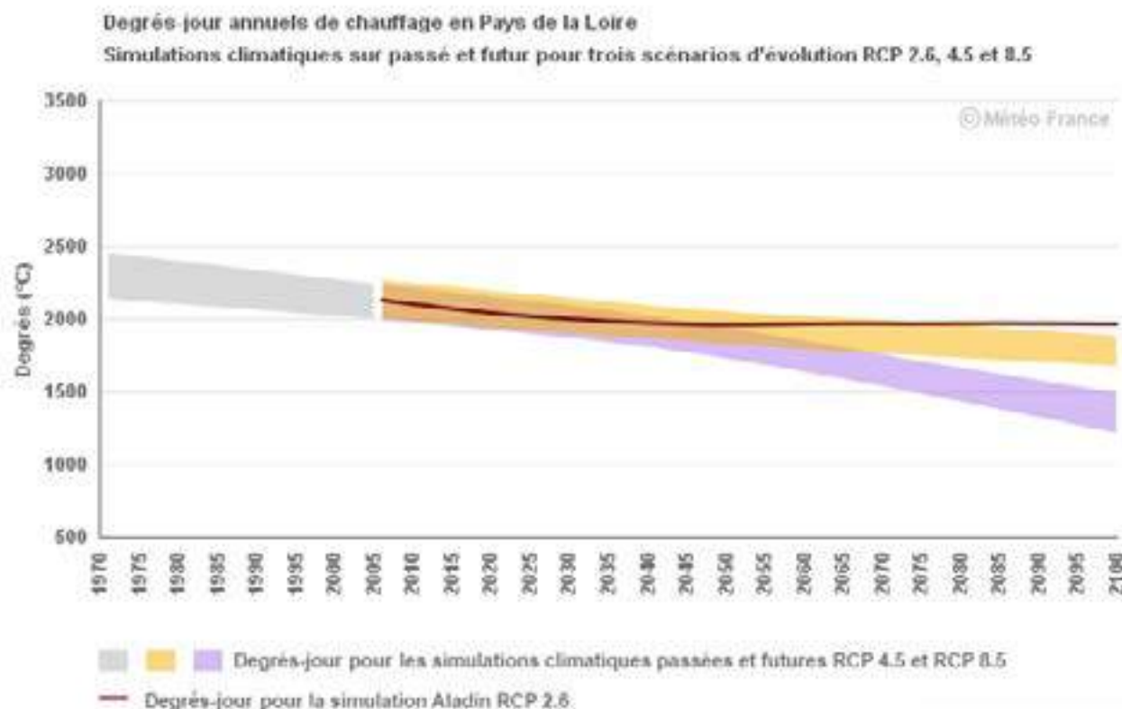
Illustration 29 : évolution des besoins en chauffage en Pays de la Loire et projection climatique. Source Climat HD Météo France
