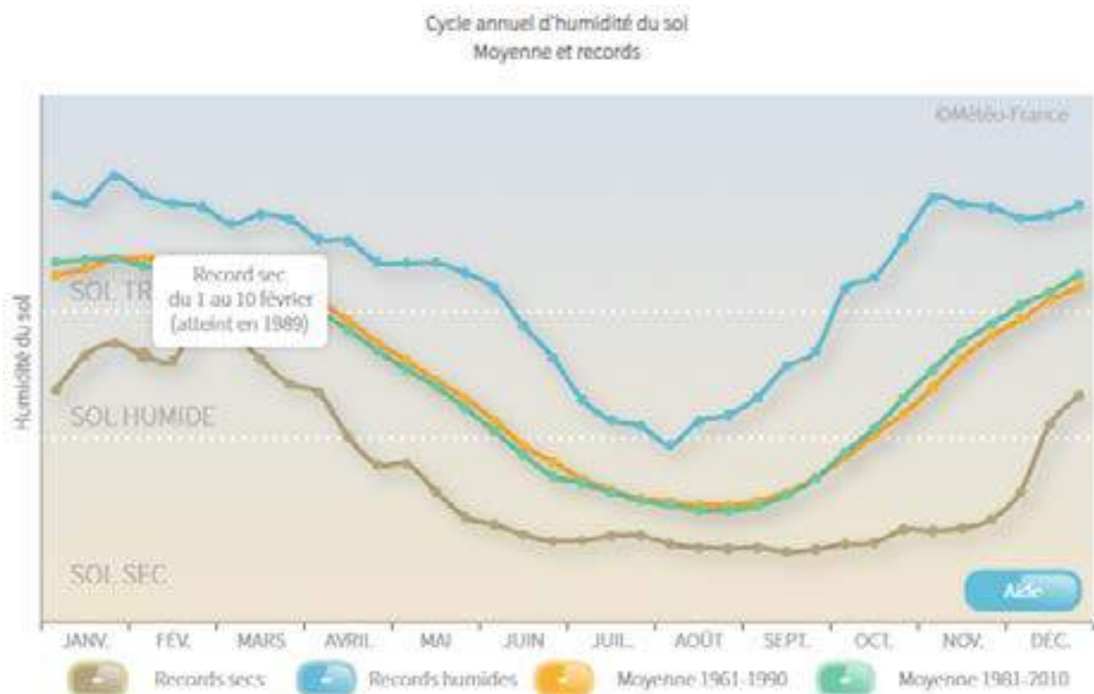
Illustration 23 : cycle annuel d'humidité des sols, moyennes et records. Source climat HD Météo France
