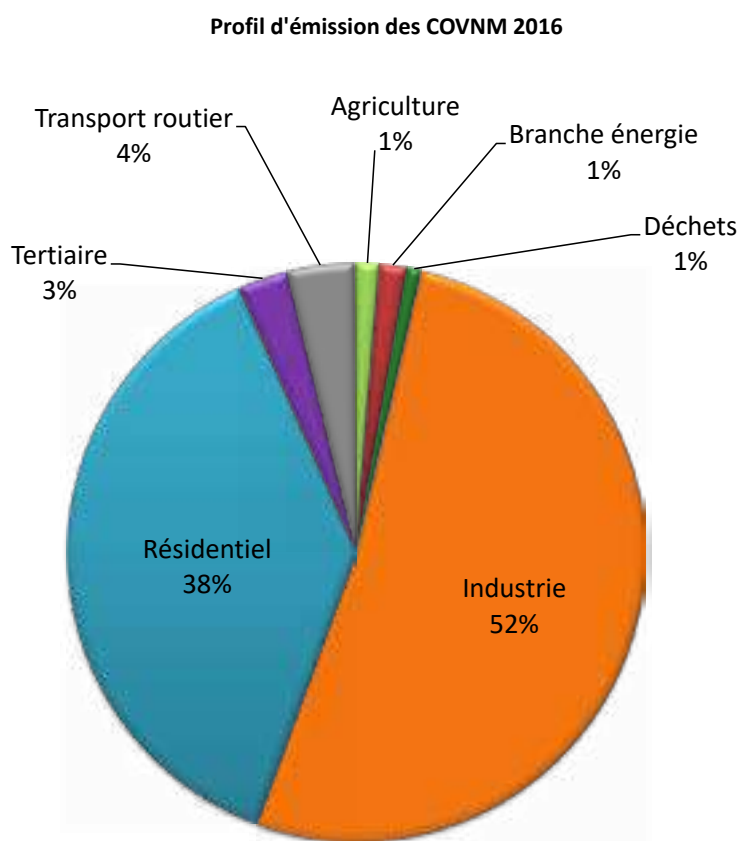
Graphique 47 : profil d'émissions des COVNM. Source données Air Pays de la Loire 2016
