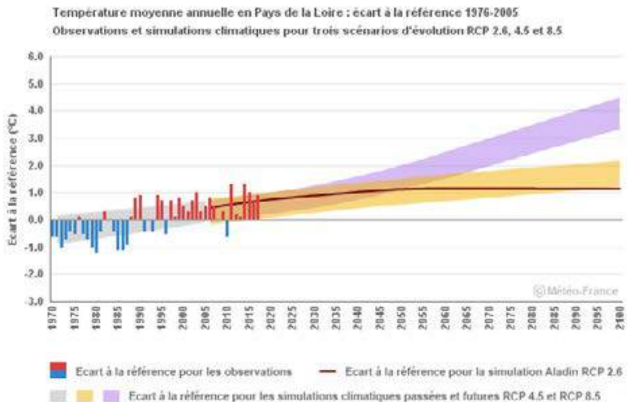
Illustration 26 : température moyenne annuelle de référence en Pays de la Loire et projections climatiques potentielles. Source : Climat HD Météo France
