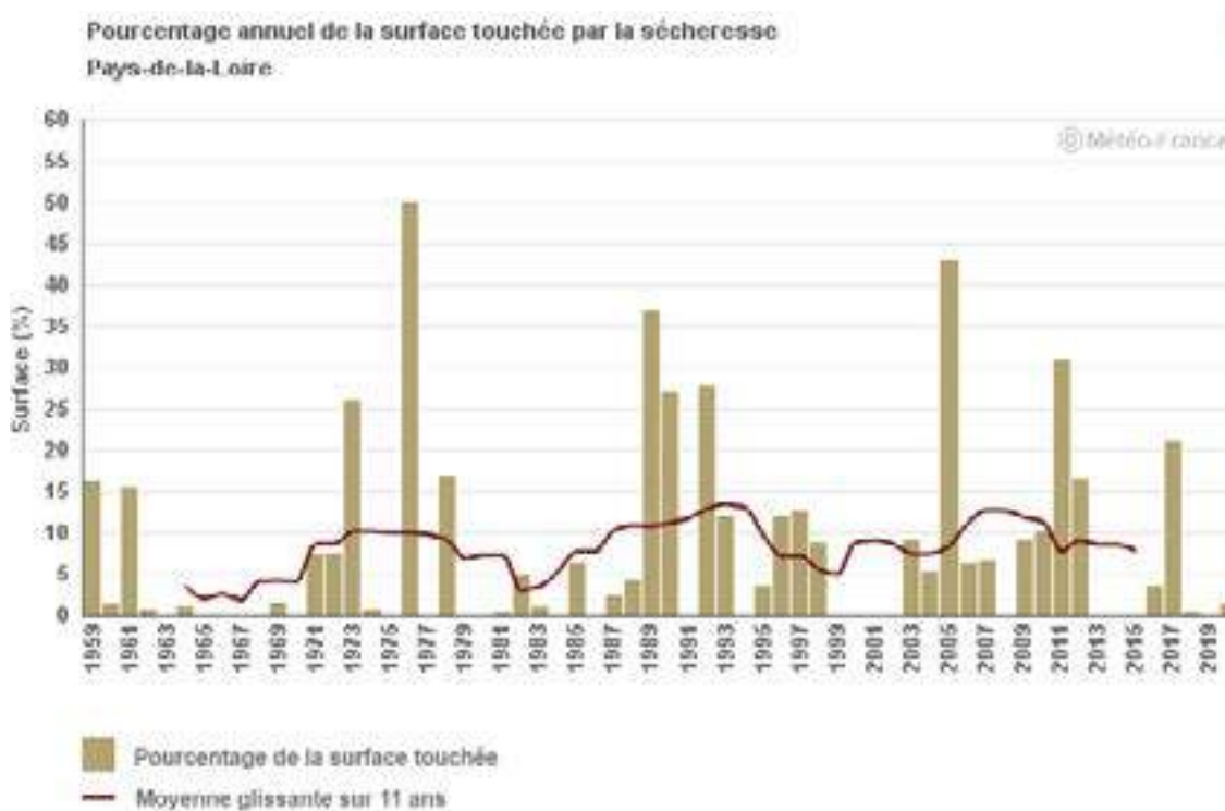
Illustration 22 : évolution de la surface de sécheresse des sols. Source climat HD Météo France
