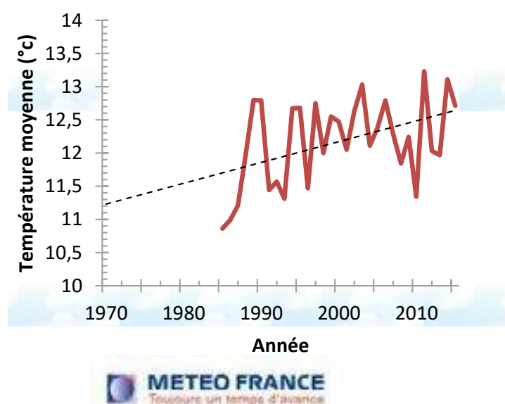
Illustration 17 : évolution des températures moyenne sur la Roche sur Yon. Source : ORACLE 2018
