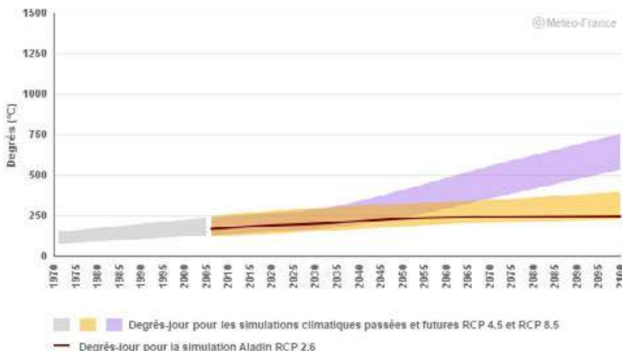
Illustration 30 : degré-jour annuel en Pays de la Loire et projection climatique. Source Climat HD Météo France
