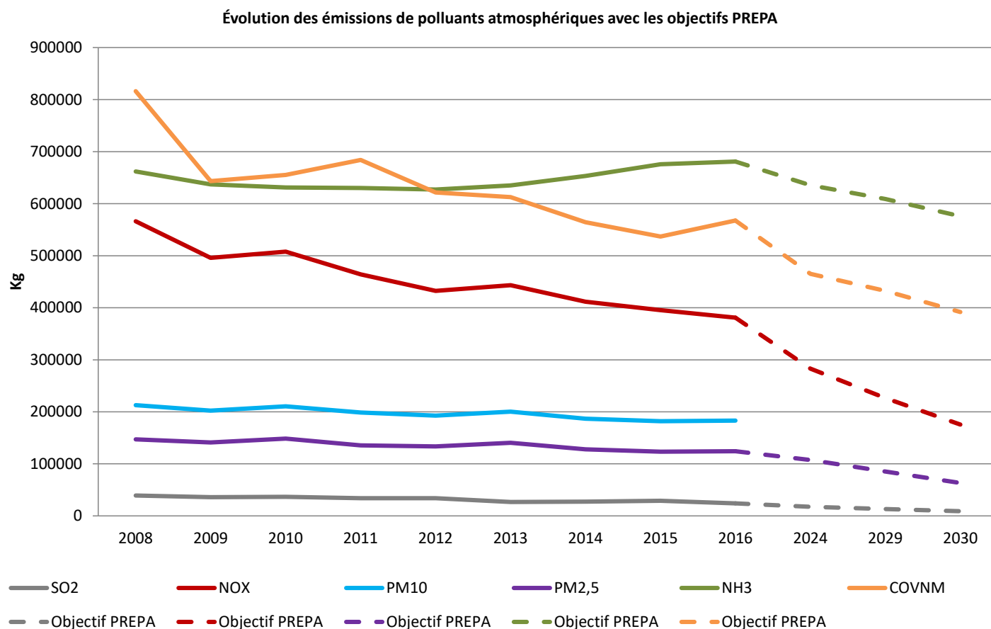
Graphique 50 : évolution des émissions de polluants atmosphériques et objectif du PREPA. Source : données Air Pays de la Loire ; PREPA
