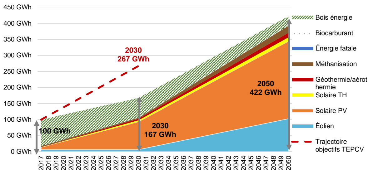
Figure 10 : Représentation graphique de la stratégie d'énergies renouvelables territoriale retenue par le Pays de Saint Gilles Croix de Vie – source : Calcul Stratégie V2207-st gilles VF.xls/EnR Calcul (2)
