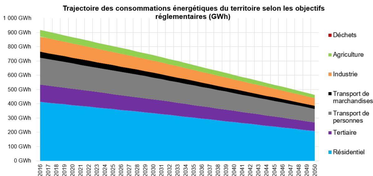
Figure 4 : Trajectoire des consommations d'énergie (en GWh) selon les objectifs nationaux sur le territoire du Pays de Saint Gilles Croix de Vie selon l'approche réglementaire – source : calcul stratégie vierge V2207-st gilles VF.xls/ conso calculs (3)
